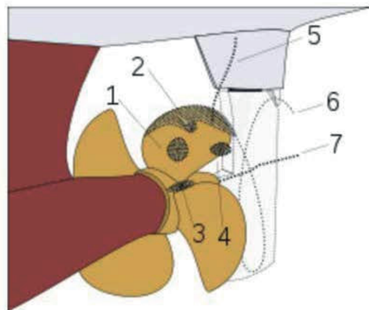
Soorten cavitatie: 1: bellen cavitatie, 2: vlies cavitatie, 3: bladwortelcavitatie, 4: vortexcavitatie, 5: schroefrompcavitatie, 6: tipwervelcavitatie, 7: naafwervelcavitatie.
